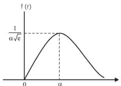
The Rayleigh PDF
